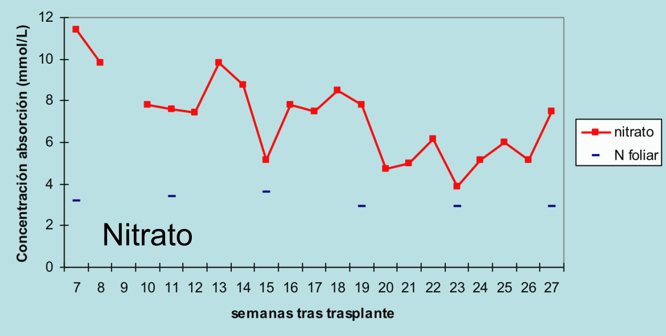
Evolución de la concentración de absorción durante el ensayo
